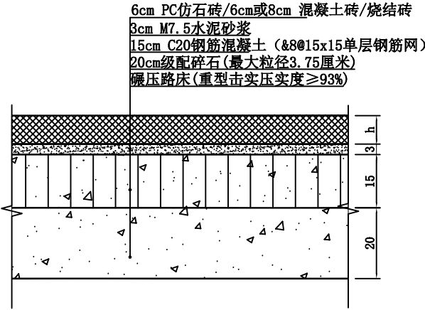
人行道翻建结构（一）
