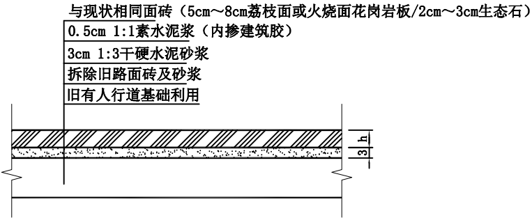
人行道换砖结构（二）
