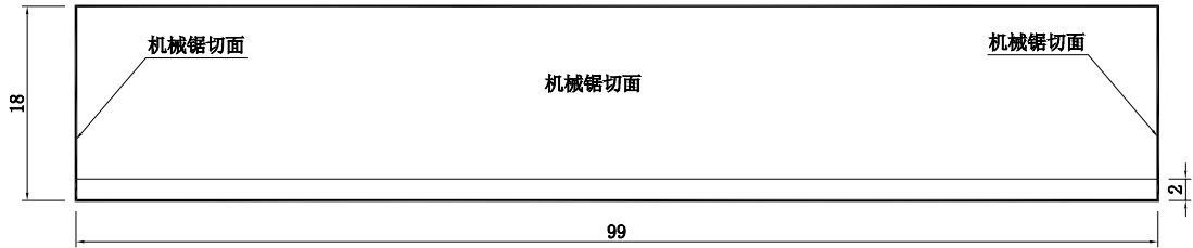
边石平面图(1:5)
