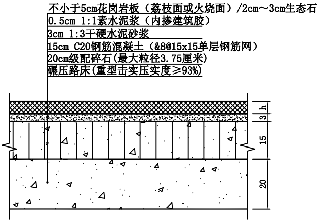
人行道翻建结构（二）
