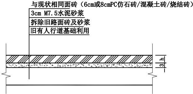
人行道换砖结构（一）
