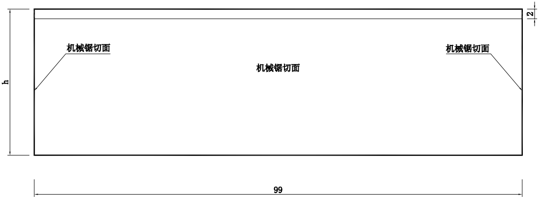
边石平面图(1:5)
