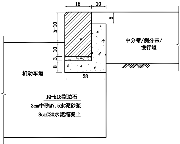
边石安装图(1:10)
