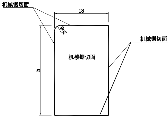
边石侧面图(1:5)
